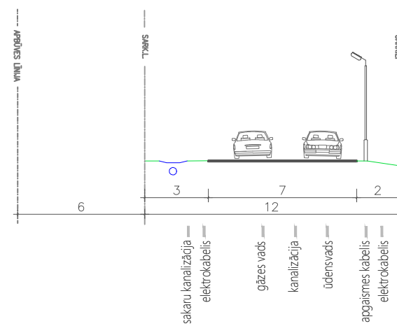
Šķēršprofils A : A 1:250
